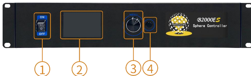
前面板
